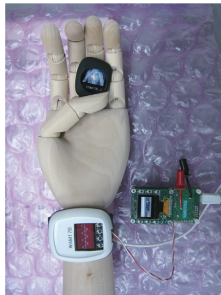
超小型・ウェアラブル計測モジュール
